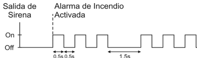
Figura 9: Salida de Sirena durante una Alarma de Fuego
