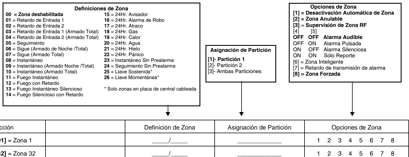
Figura 8: Programación de Zonas
