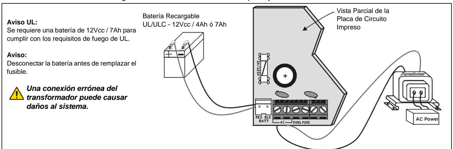
Figura 1: Conexiones de Batería de Respaldo y de Alimentación CA
