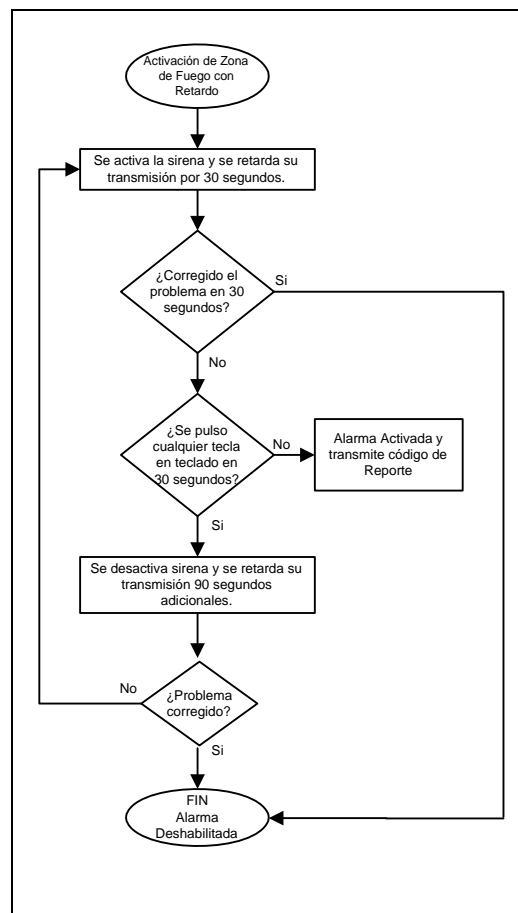
Figura 10: Zona de Fuego Retardado de 24hrs
