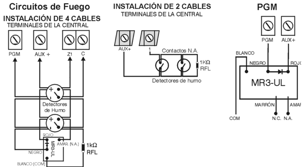
Figura 5: Circuitos de Fuego
