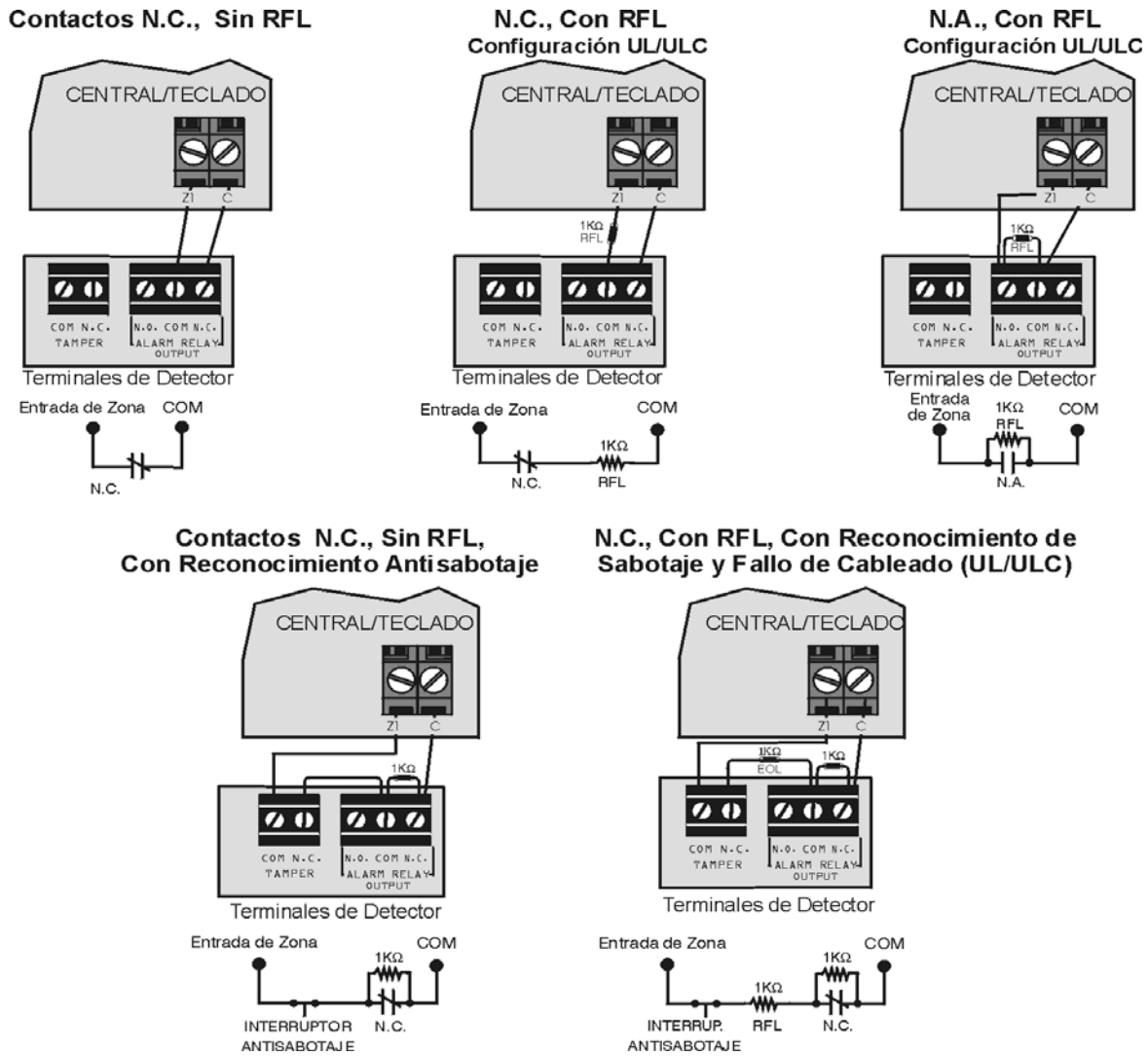
Figura 3: Conexiones de Entrada de Zona Simple
