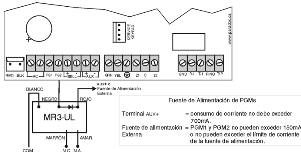
Figura 2: Conexiones de Relé y de PGM
