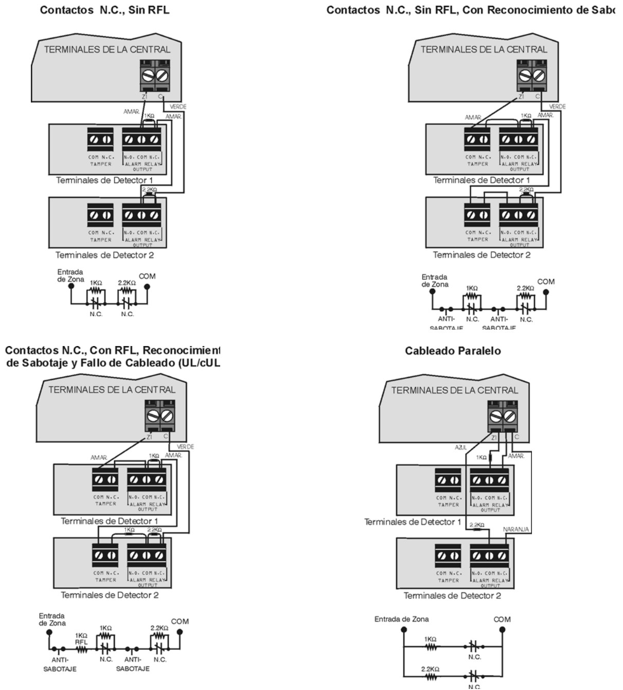
Figura 4: Conexiones de Zona de Tecnología Avanzada
