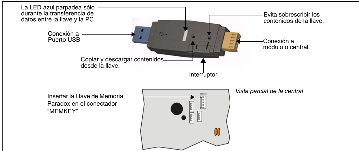
Figura 7: Llave de Memoria Paradox
