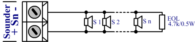
Fig. 3 - Conexión de sirenas a la salida S_n
